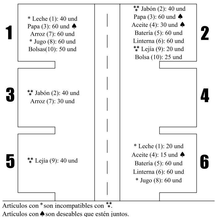
Figura 4.4: Distribución óptima de productos en los muelles.
